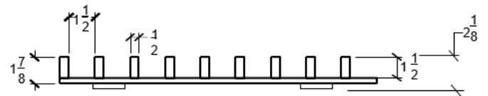
1 1/2" Cambio Rainier Fins Panel
